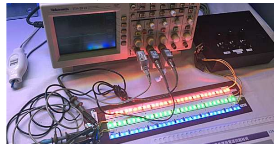
PWM/定電流調光比較デモ
